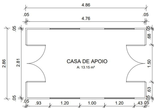
1 CASA DE APOIO - PLANTA BAIXA ATUAL ESC: 1/50
