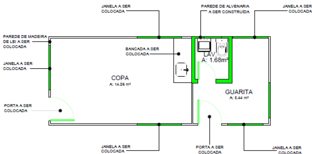
2 CASA DE APOIO - PLANTA DE CONSTRUIR ESC: 1/50
